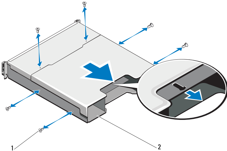
Abbildung 16-15. Entfernen und Installieren des RAID-Controller-Moduls/Netzteilgehäuses
