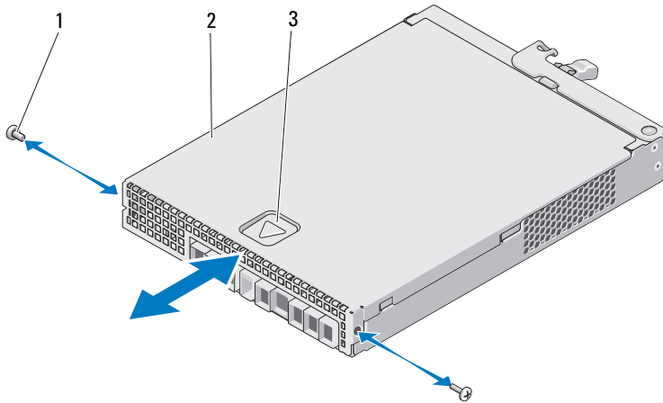
Abbildung 16-9. Öffnen und schließen des RAID-Controller-Moduls
