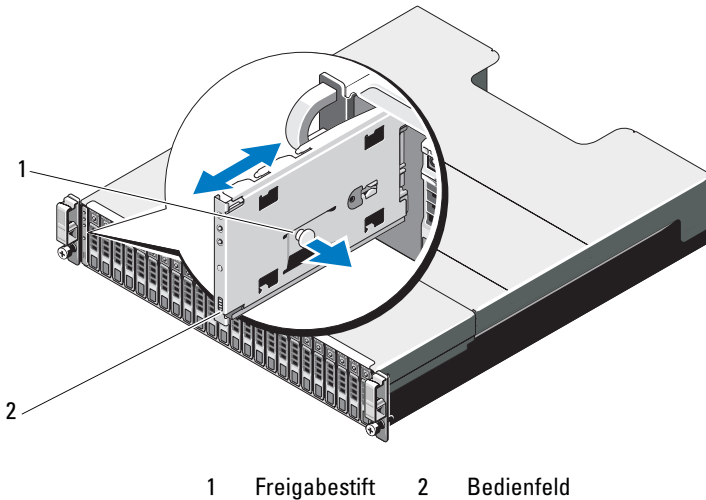
Abbildung 16-14. Entfernen und Installieren der Bedienfeldplatine – PowerVault MD3620f
