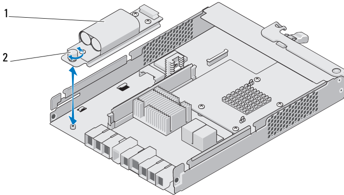
1 Akkusicherungsmodul 2 Schraube
