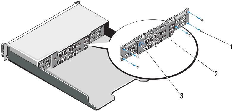
Abbildung 16-16. Entfernen und Installieren der Rückwandplatte – PowerVault MD3600f
