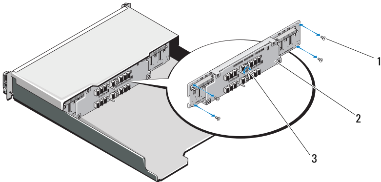
Abbildung 16-17. Entfernen und Installieren der Rückwandplatte – PowerVault MD3620f
