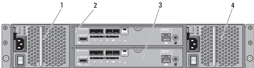
Abbildung 2-4. Funktionen und Anzeigen auf der Rückseite–Dell PowerVault MDMD3600f-Serie
