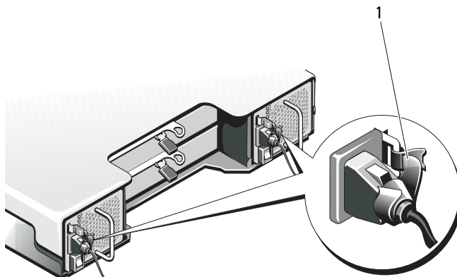
Abbildung 16-12. Sichern des Netzstromkabels
