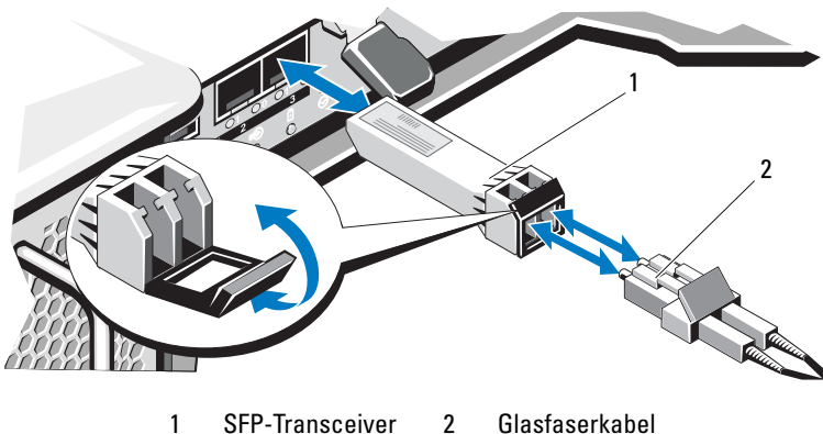
Abbildung 3-2. Glasfaserkabelverbindung
