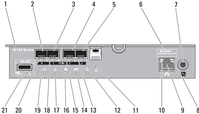
Abbildung 3-1. RAID-Controller-Modul für MD3600f Series Fibre Channel
