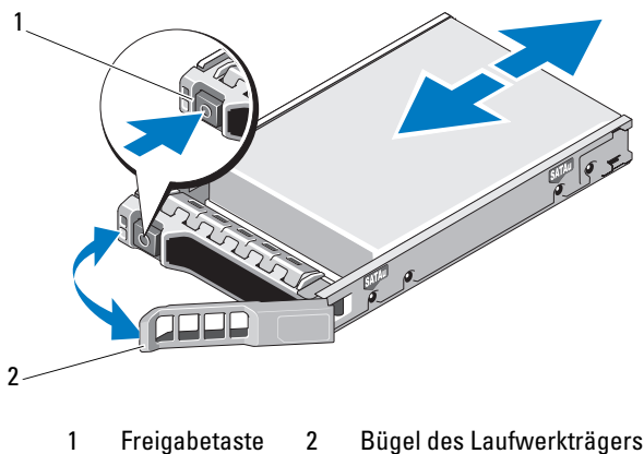
Abbildung 16-4. Laufwerk entfernen und installieren
