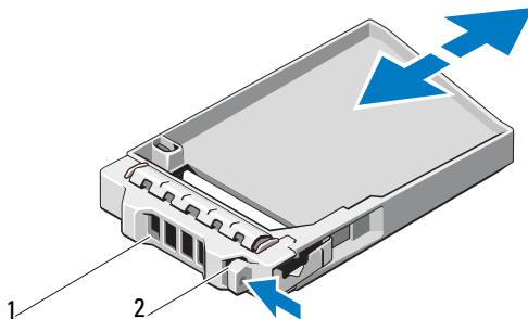
Abbildung 16-3. Entfernen und Installieren eines 2,5-Zoll-Laufwerkplatzhalters (Nur MD3620f)
