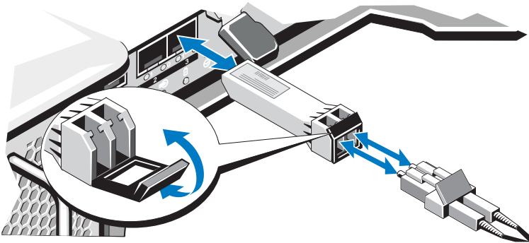
Abbildung 20-1. Entfernen eines SFP-Moduls
