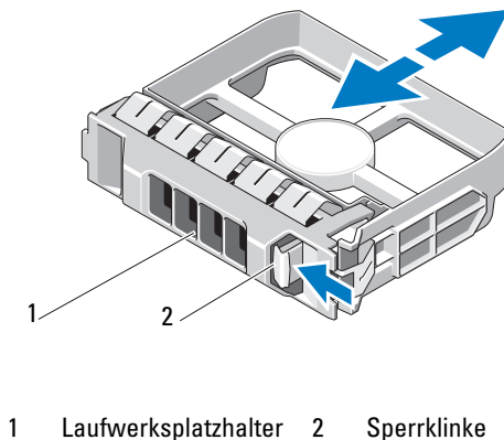
Abbildung 16-2. Entfernen und Installieren eines 3,5-Zoll-Laufwerkplatzhalters (Nur MD3600f)
