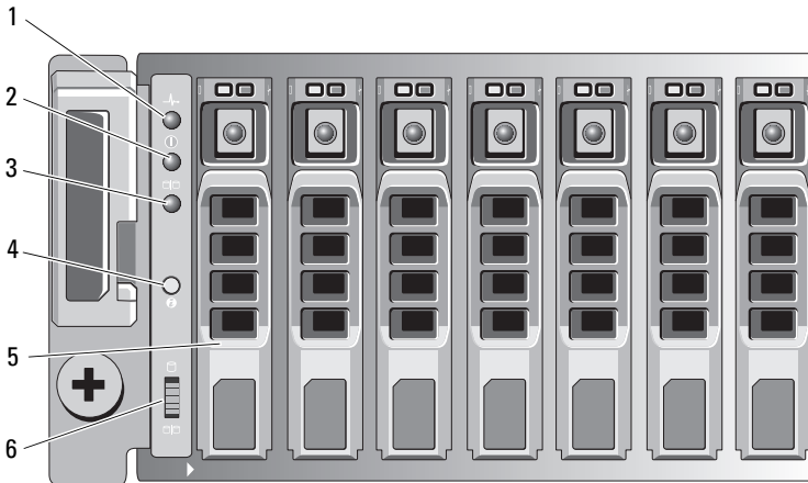
Abbildung 2-2. Funktionen und Anzeigen auf der Vorderseite – Dell PowerVault MD3620f
