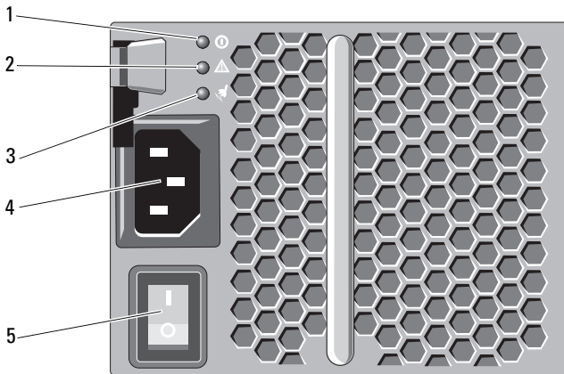
Abbildung 2-6. Anzeigecodes und Funktionen für Stromversorgung
